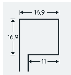
ΘΕΡΜΟΜΟΝΩΤΙΚΟ ΣΥΝΘΕΤΙΚΟ ΚΟΥΤΙ ΕΠΙΚΑΘΗΜΕΝΟ T16.9 ME feliblok plus
