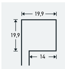
ΘΕΡΜΟΜΟΝΩΤΙΚΟ ΣΥΝΘΕΤΙΚΟ ΚΟΥΤΙ BASIC ΕΠΙΚΑΘΗΜΕΝΟ T19.9
